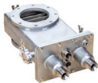
ЛАП-100П АЗОТНАЯ ПРОТОЧНАЯ ВАКУУМНАЯ ЛОВУШКА
