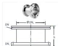
Адаптеры ISO-K / CF Материал исполнения: нержавеющая сталь
